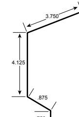
9. Fascia/Eave Trim
