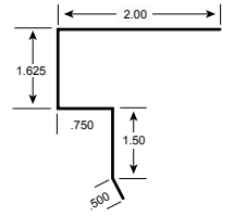
5. Rake Trim
