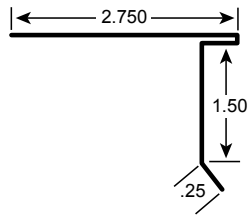
7. Drip Edge
